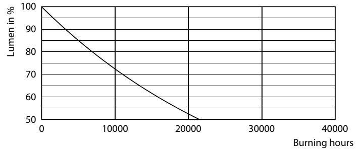
Lumen Maintenance Diagram - 11A19/LED/827/FR/P/ND 4/4FB
