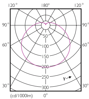
Light Distribution Diagram - 14A19/LED/827/FR/P/ND 4/2FB
