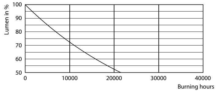
Lumen Maintenance Diagram - 14A19/LED/827/FR/P/ND 4/4FB
