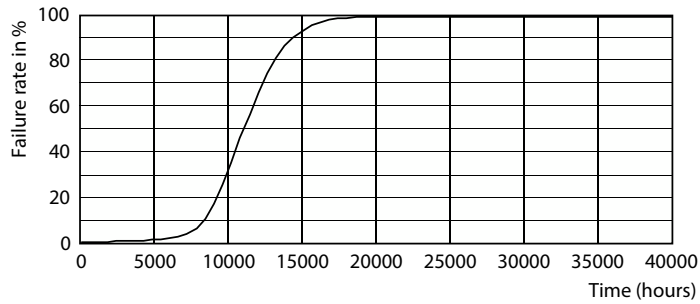
Life Expectancy Diagram - 5.5A19/LED/850/FR/P/ND 4/2FB
