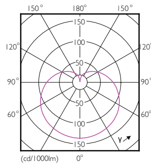
Light Distribution Diagram - 5.5A19/LED/850/FR/P/ND 4/2FB
