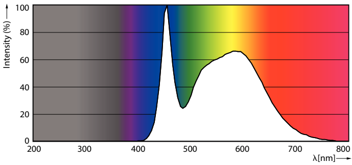
LedBulb A19 E26 7W 850
