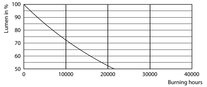
Lumen Maintenance Diagram - 10A19/LED/850/FR/P/ND 4/4FB
