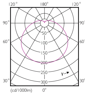
Light Distribution Diagram - 10A19/LED/850/FR/P/ND 4/4FB
